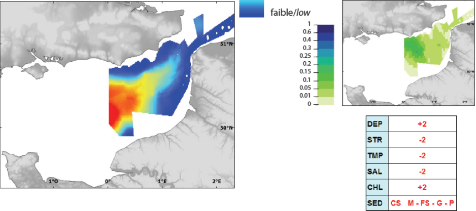
Habitat potentiel en janvier (RQ) Potential habitat in January (RQ)
