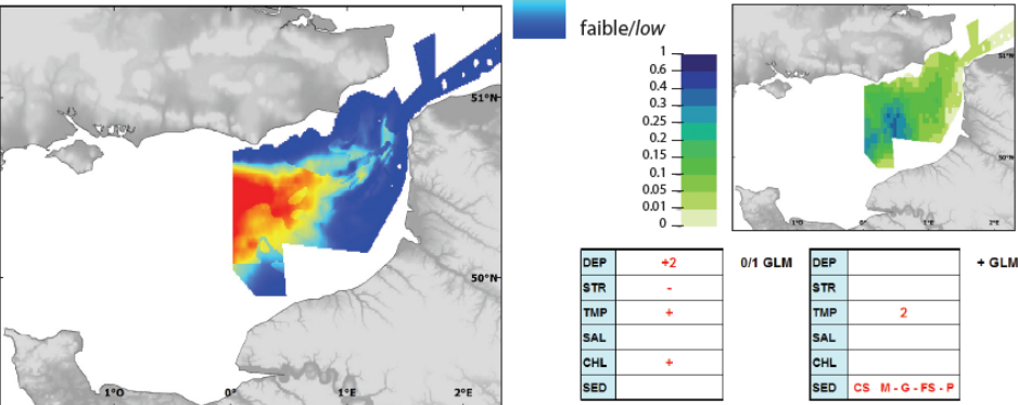
Habitat potentiel en janvier (RQ) Potential habitat in January (RQ)
