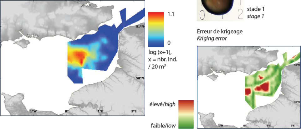
Abondance en janvier (IBTS, 2007) Abundance in January (IBTS, 2007)
