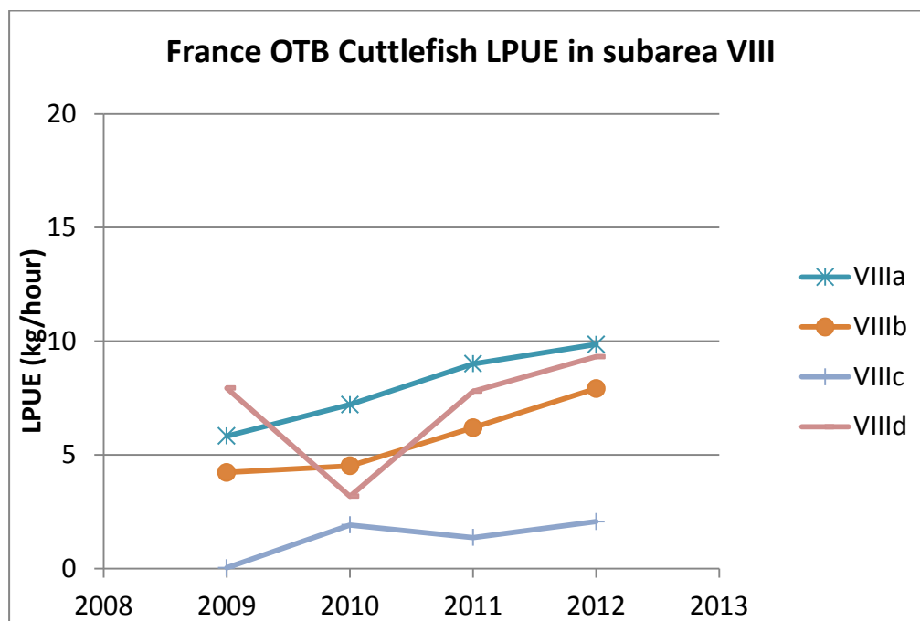
Figure 3.1.3.1.4.1. Sepiidae LPUEs (kg/h) for French Otter Bottom Trawl in Subarea VIII in 2009-2012.
